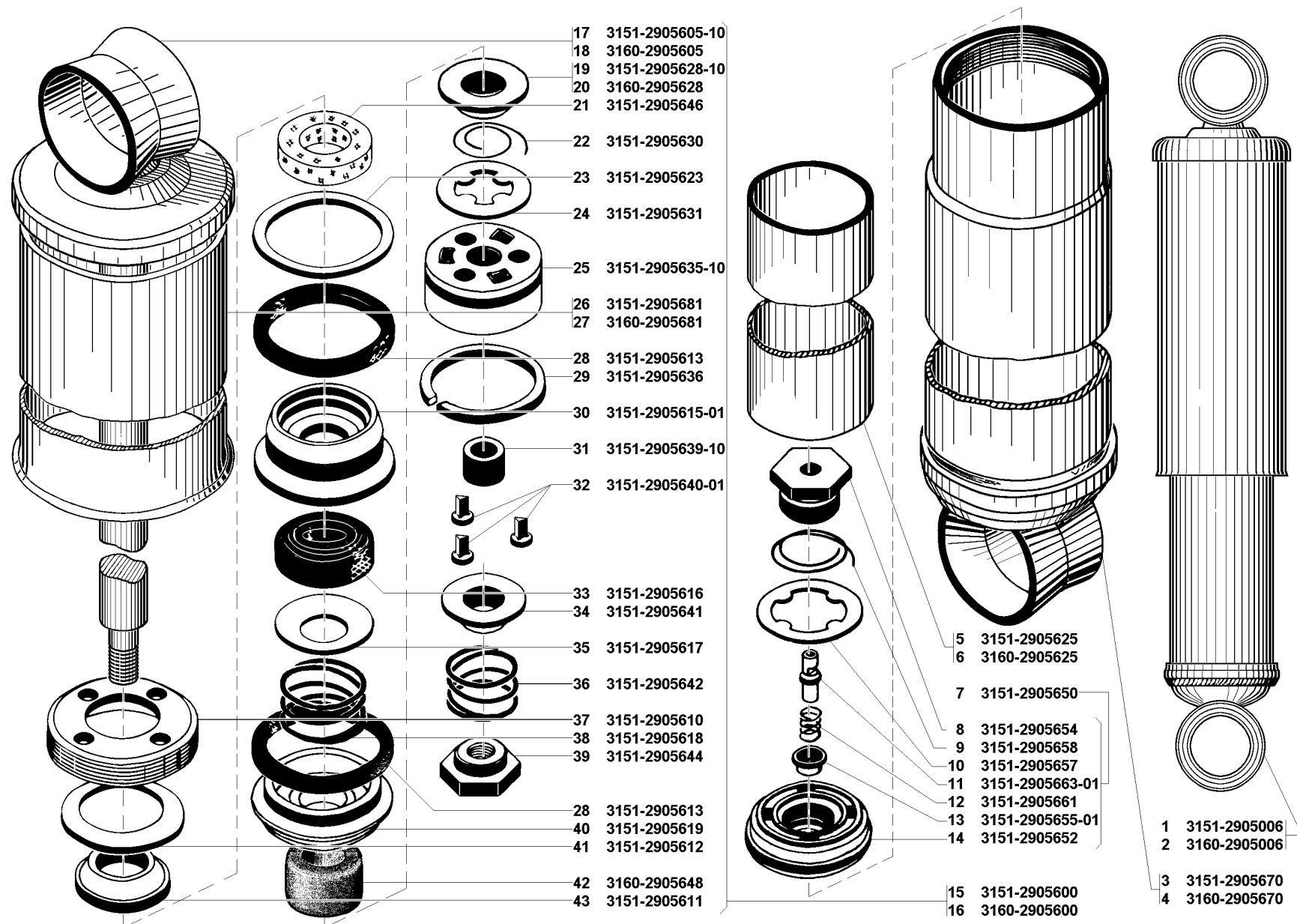
Рис. 85. Амортизаторы передние (2905)/1
