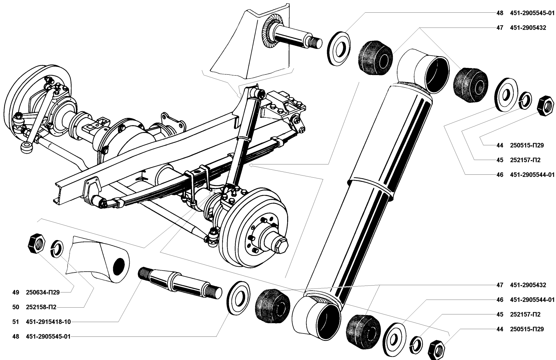
Рис. 86. Амортизаторы передние (2905)/2
